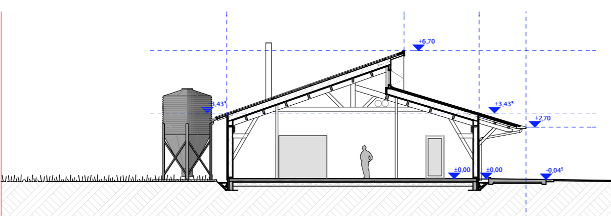
COUPE SUR TERRAIN
