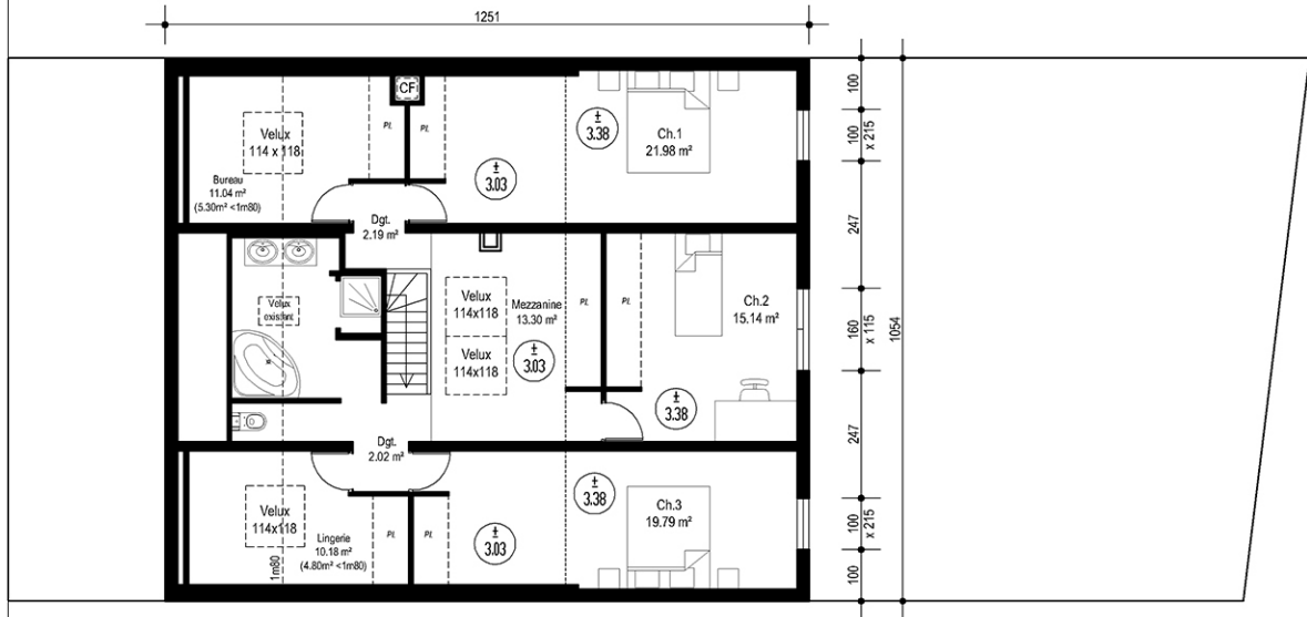
Plan Projet Etage 1/100ème
