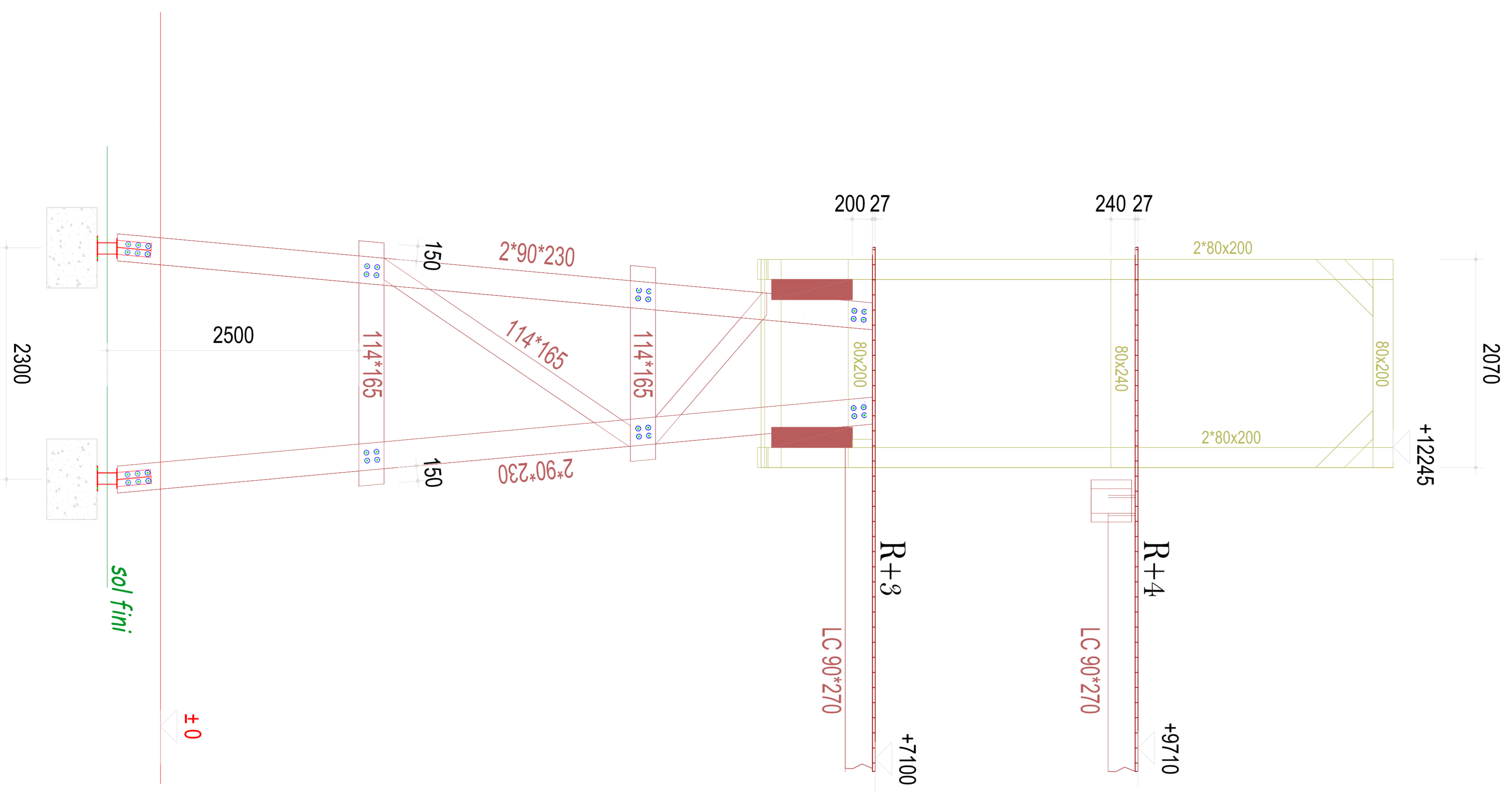
Coupe B-B
