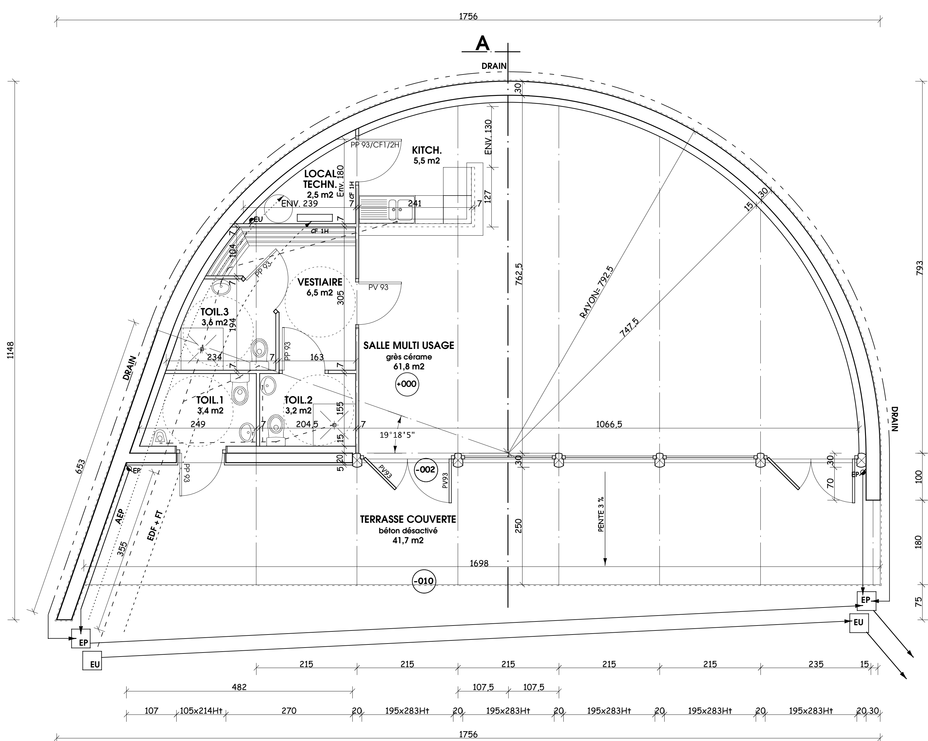
PLAN Niveau 0 1/50 000 = 874,70
